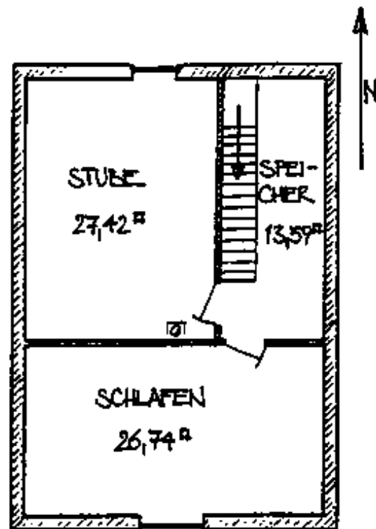
DACHGESCHOSS
