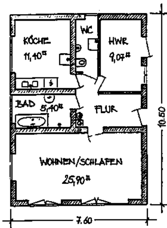
ERDGESCHOSS M:1:100
